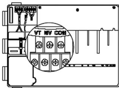
Zawory Stacyjne
